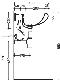
sezione longitudinale / section
